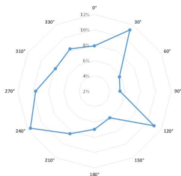
Figure 6 : Rose des vents du site d'études (source : Nordex, 2019)
