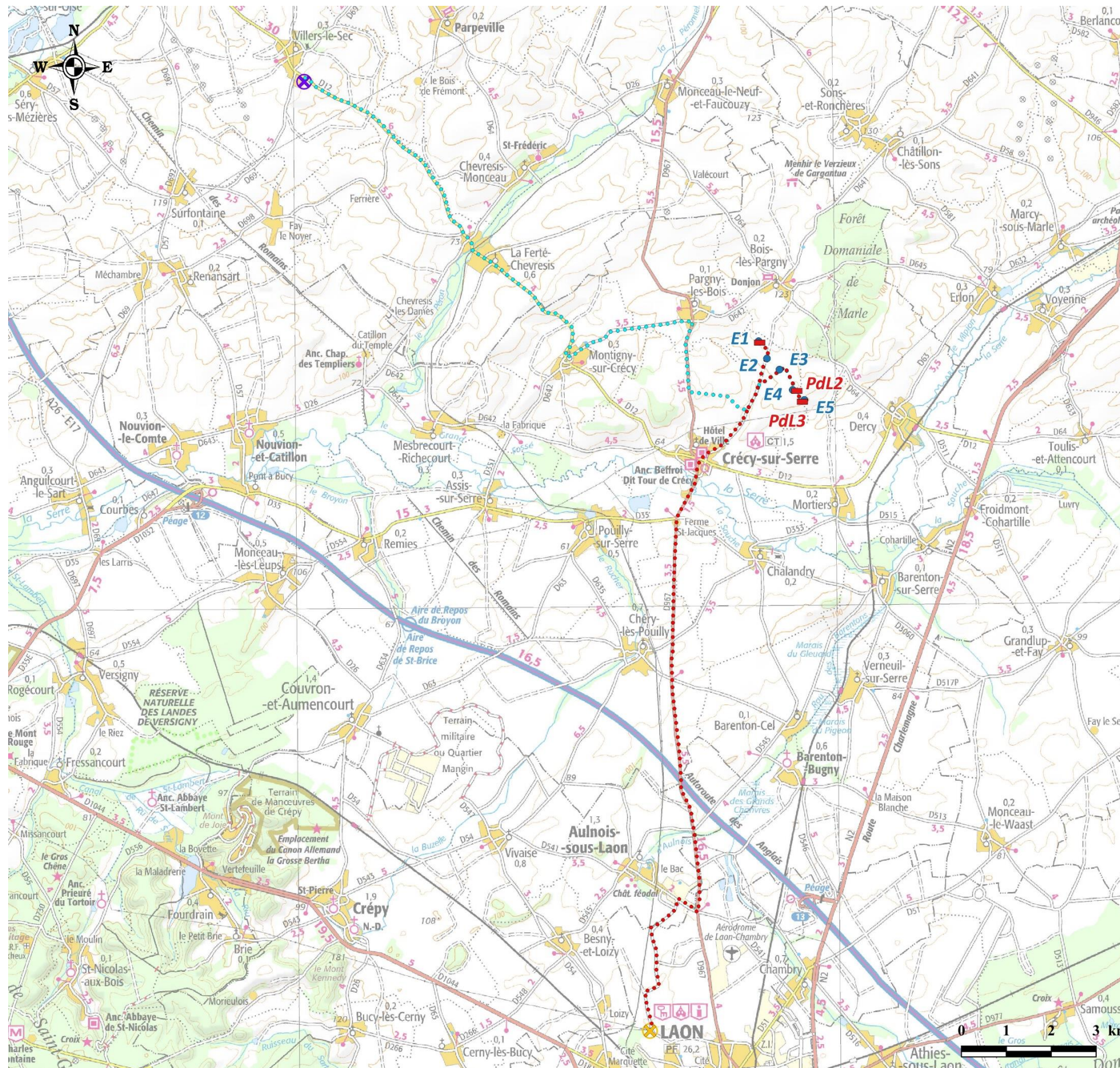
Carte 16 : Tracé provisoire du raccordement du parc éolien du Chemin Vert au réseau public de transport d'électricité
