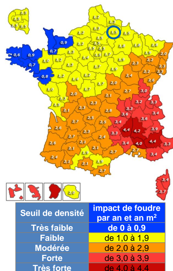
Carte 10 : Densité de foudroiement – Cercle bleu : Périmètre d'étude de dangers (source : Météo Paris, 2019)
