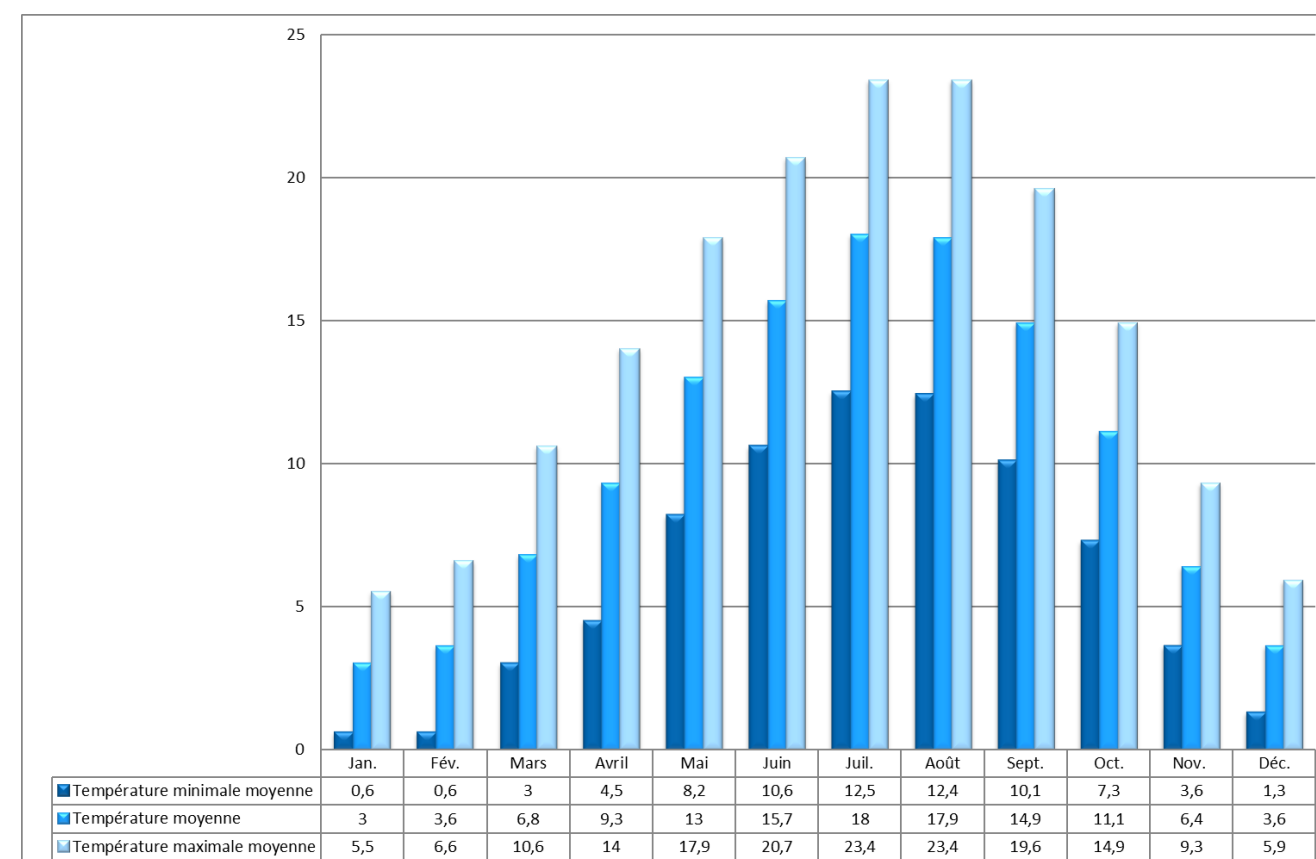
Figure 4 : Illustration des températures de 1981 à 2010 – Station de Saint-Quentin Roupy (source : Infoclimat.fr, 2019)
