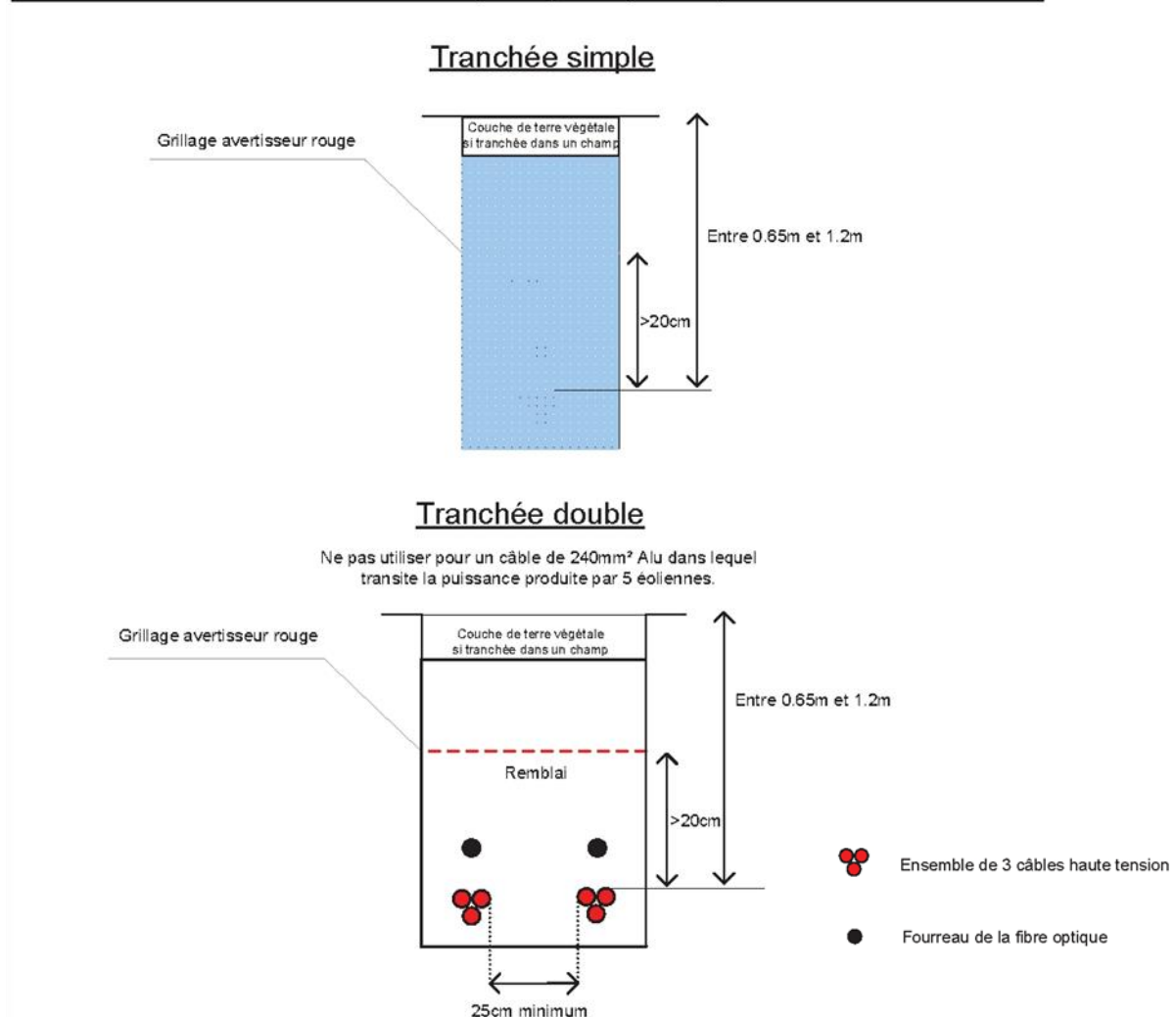
Figure 11 : Coupes-types de tranchées (source : Nordex, 2019)
