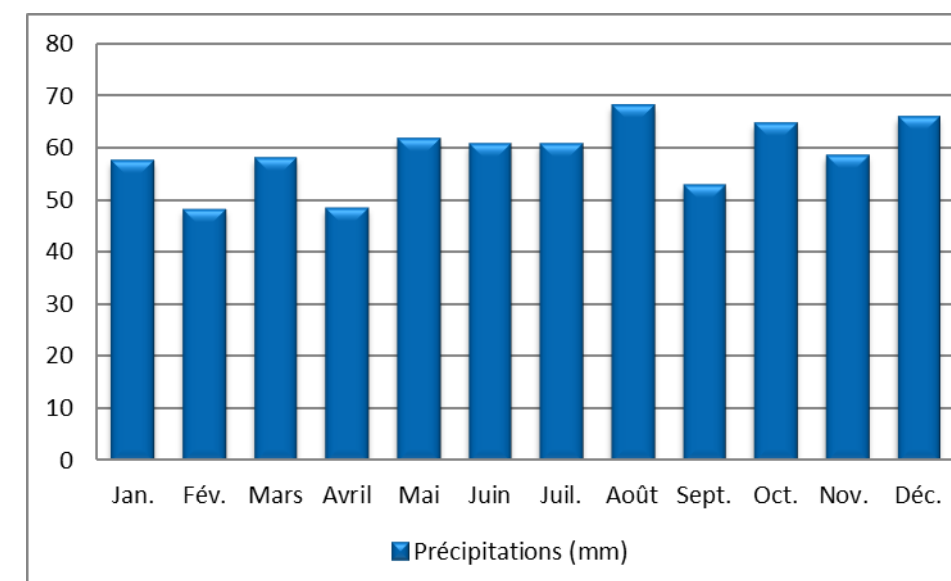
Figure 5 : Illustration des précipitations de 1981 à 2010 – Station de Saint-Quentin Roupy (source : Infoclimat, 2019)
