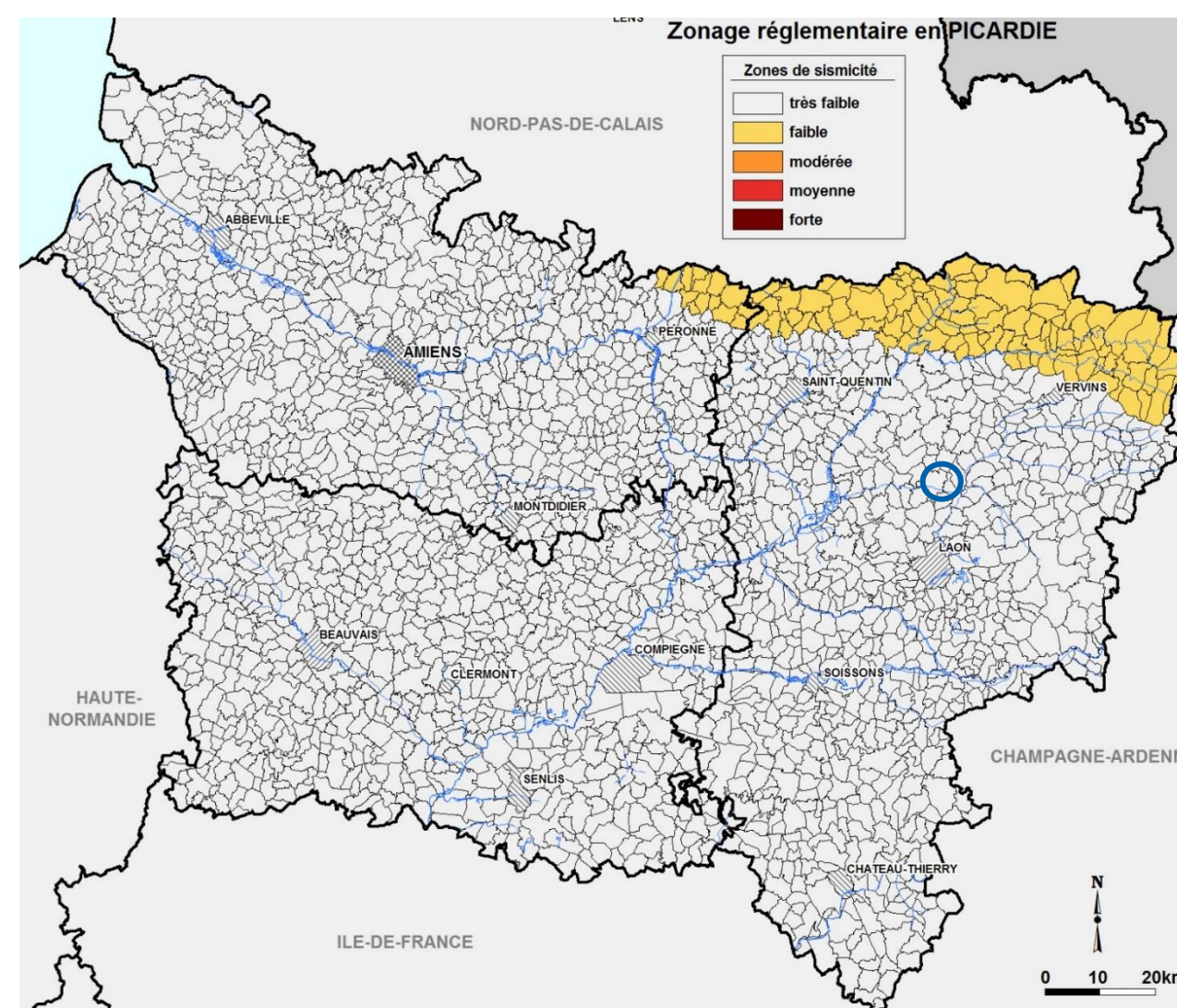
Carte 9 : Zonage sismique de l'ancienne région Picardie – Cercle bleu : Périmètre d'étude de dangers (source : planseisme.fr, 2015)
